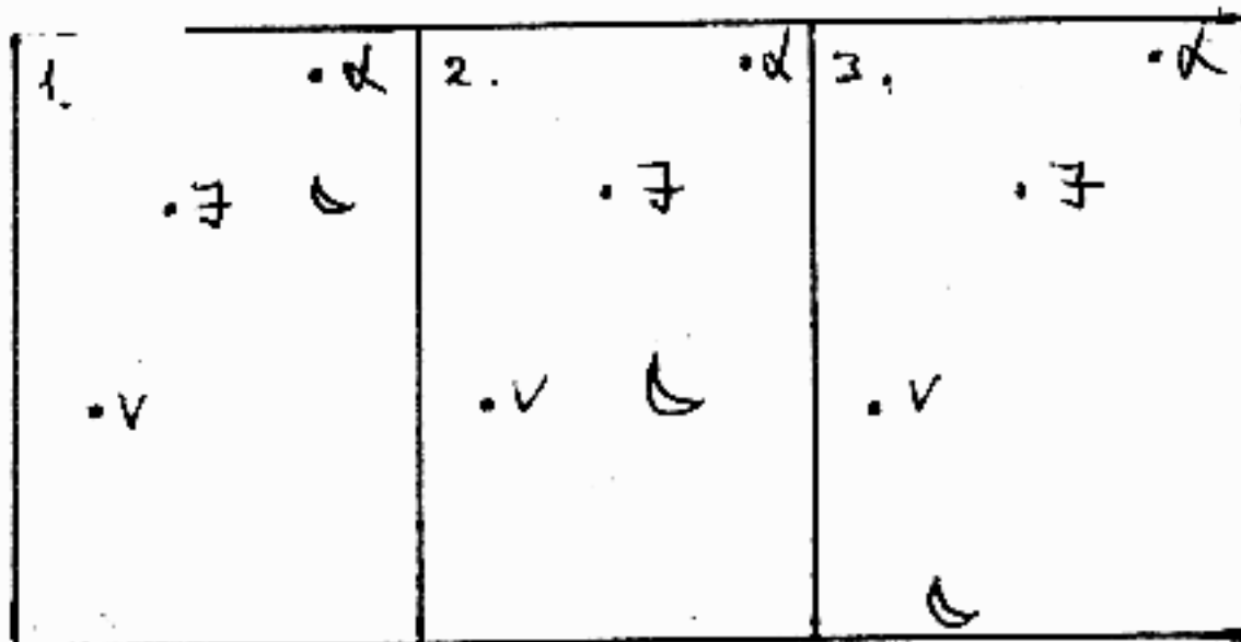
Vénusz - Jupiter - Regulus - Hold együttállás a hajnali égen /nov.1-3./
